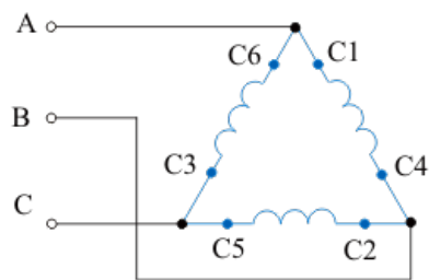
Схема включения обмоток двигателя
