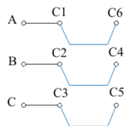
Схема включения обмоток двигателя
