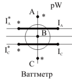
Обозначение выводов обмоток приборов
