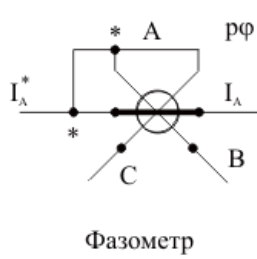
Обозначение выводов обмоток приборов
